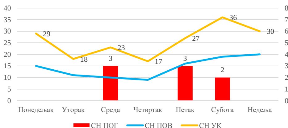
Графикон 7.4. Број саобраћајних незгода по данима у недељи, за период од 2019. до 2023. године.
