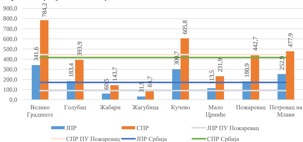
Графикон 10.3. Упоредна анализа јавног пондерисаног и саобраћајног пондерисаног ризика страдања у саобраћају у односу на ПУ Пожаревац и Републику Србију, током 2022. године.
