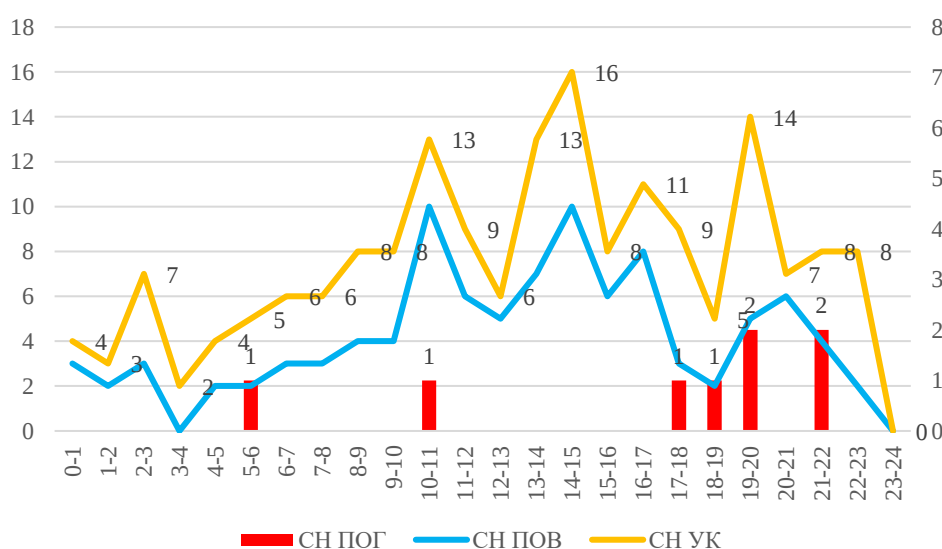
Графикон 7.5. Број саобраћајних незгода по часовима у дану, за период од 2019. до 2023. године.
