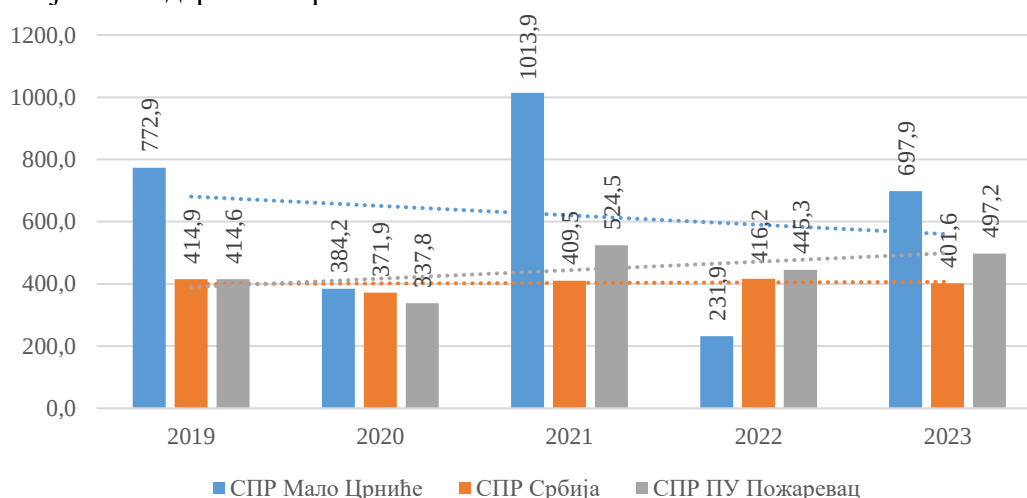
Графикон 10.2. Саобраћајни пондерисани ризик страдања у саобраћајним незгодама, за период од 2021. до 2023. године.
